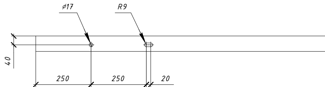
Поз. 1 (1:10)
