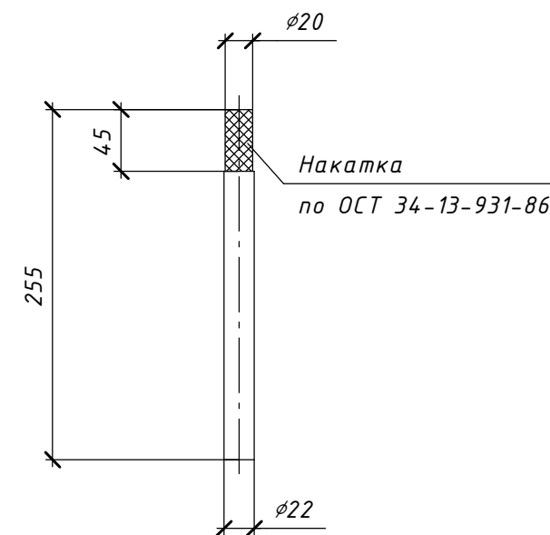
Поз. 4 (1:5)
