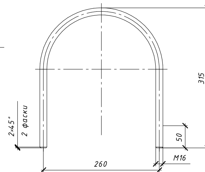
Поз. 5 (1:5)
